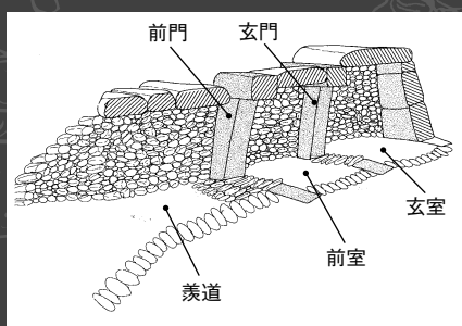
「遠見塚古墳」(旧、三番塚古墳)石室復元図
